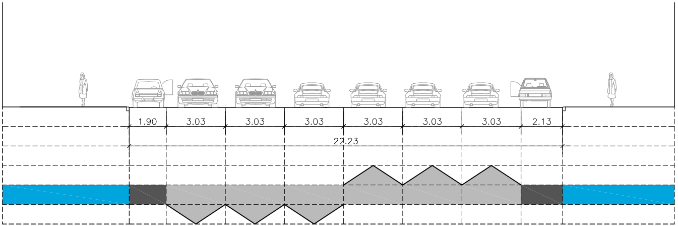
SECCIÓN S1.32 ESTADO ACTUAL
