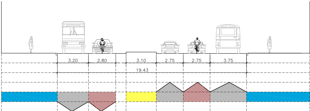
SECCIÓN S1.2 ESTADO REFORMADO
