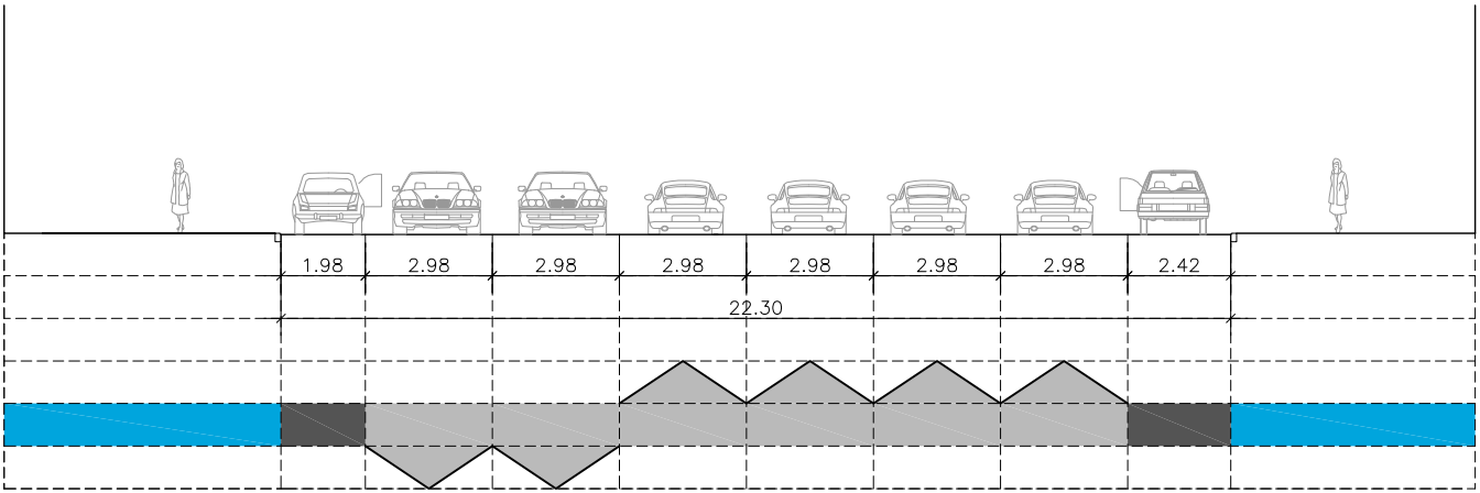
SECCIÓN S1.31 ESTADO ACTUAL
