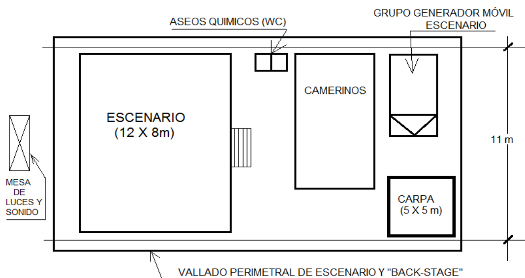
③ PLANO DETALLE ESCENARIO Y "BACK-STAGE" FIESTAS 2014
